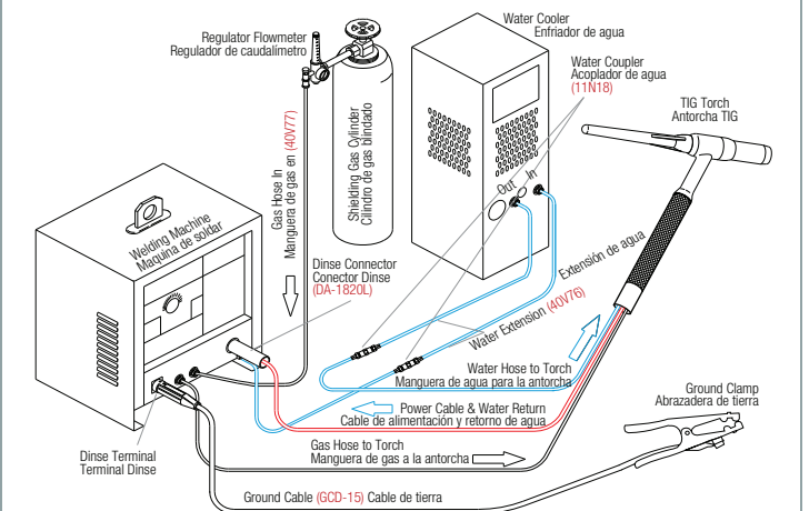
For Machines with Dinse Connectors and Gas Solenoid Using City water Para maquinas con solenoid de gas y conectores Dinse Usando agua de la ciudad
