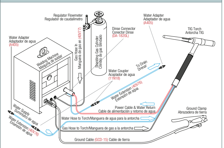
For Machines with Dinse Connectors and Gas Solenoid Using City water Para maquinas con solenoid de gas y conectores Dinse Usando agua de la ciudad
