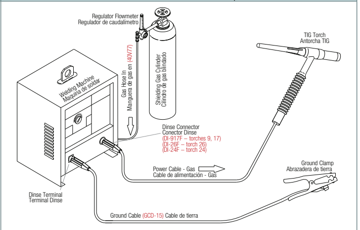
For Machine Equipped With In-line Dinse Connector Torch without Valve, 1 Piece Power Cable Para maquinas con solenoid de gas y conectores Dinse para del pase flujo, Antorcha sin válvula, cable de alimentación una pieza
