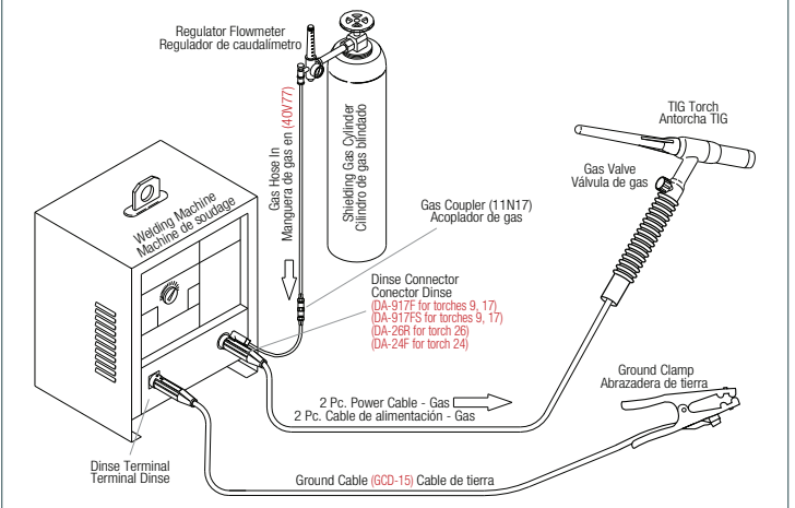
For Machine With Dinse Connector Without Gas Solenoid Torch with Valve, 2 Piece Power Cable Para maquinas sin solenoid de gas y montages usando conectores dinse Antorcha con válvula, cable de alimentación dos piezas
