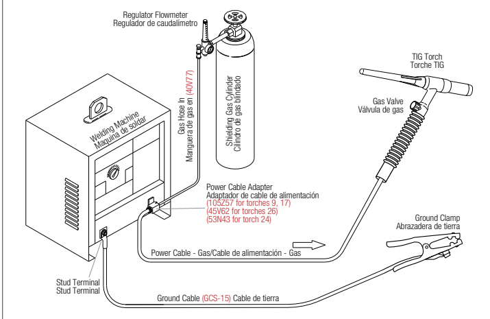
For Stud Machine Without Gas Solenoid Torch with Valve, 2 Piece Power Cable Para maquinas sin solenoid de gas y montages terminales Antorcha con válvula, cable de alimentación dos piezas
