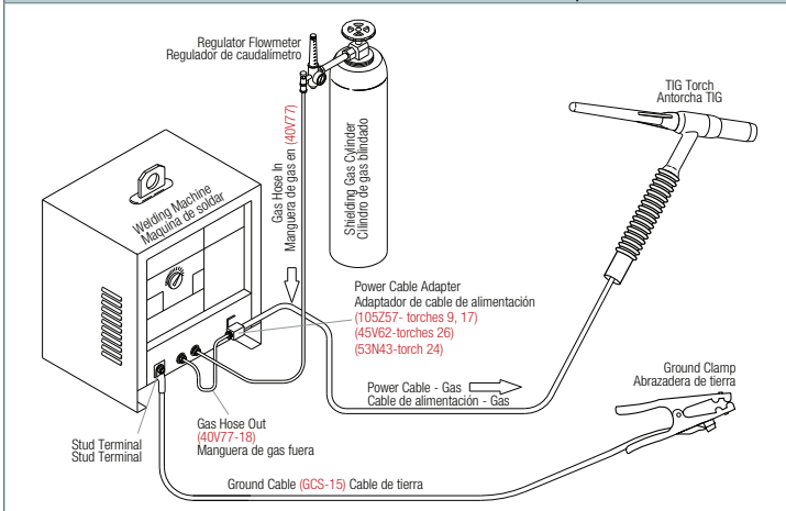
For Stud Machine With Gas Solenoid Torch without Valve, 1 Piece Power Cable Para maquinas con solenoid de gas y montages terminales Antorcha sin válvula, cable de alimentación una pieza
