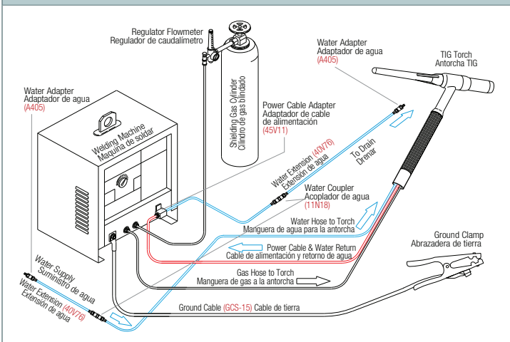
For Stud Machines With Gas Solenoid Using City Water Para maquinas con solenoid de gas y montajes terminales Usando agua de la ciudad
